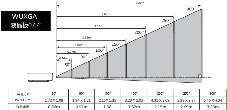
投射距离表 0.5
